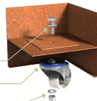
ROUE
